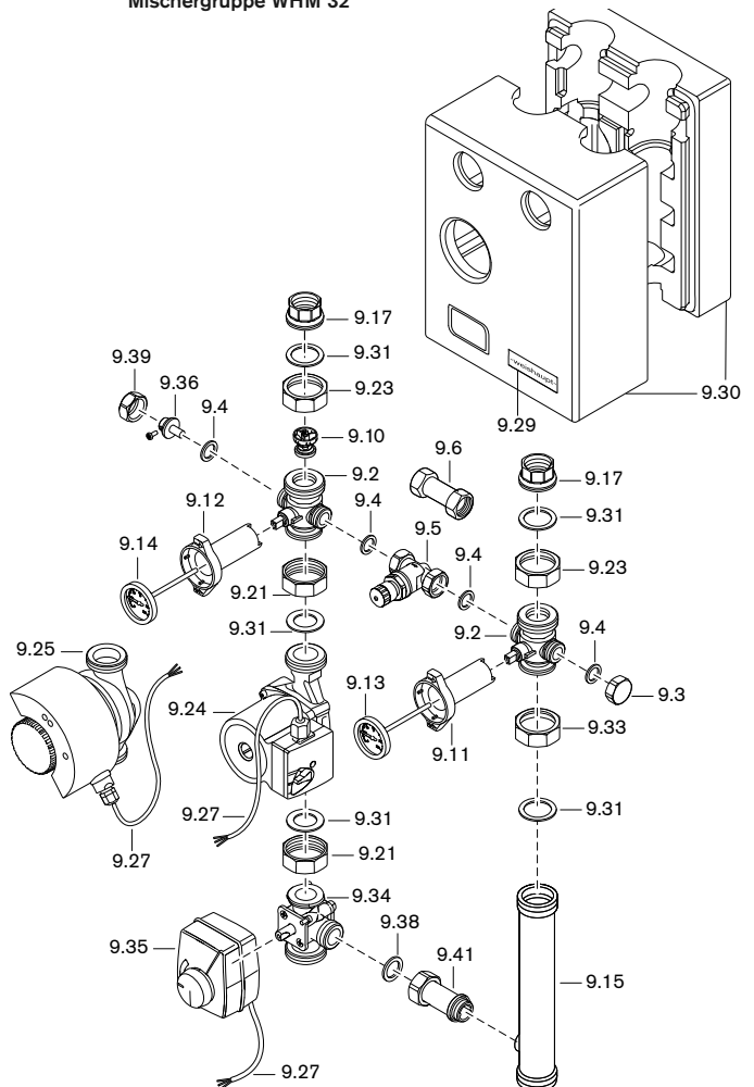
Mischerguppe WHM 32
