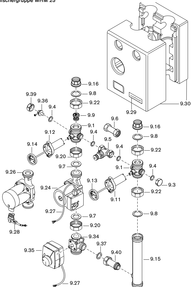
Mischerguppe WHM 25
