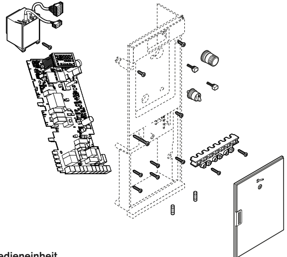
Bedieneinheit
