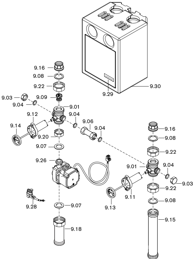
Mischergruppe / mixer assembly / groupes de mélange NW25
