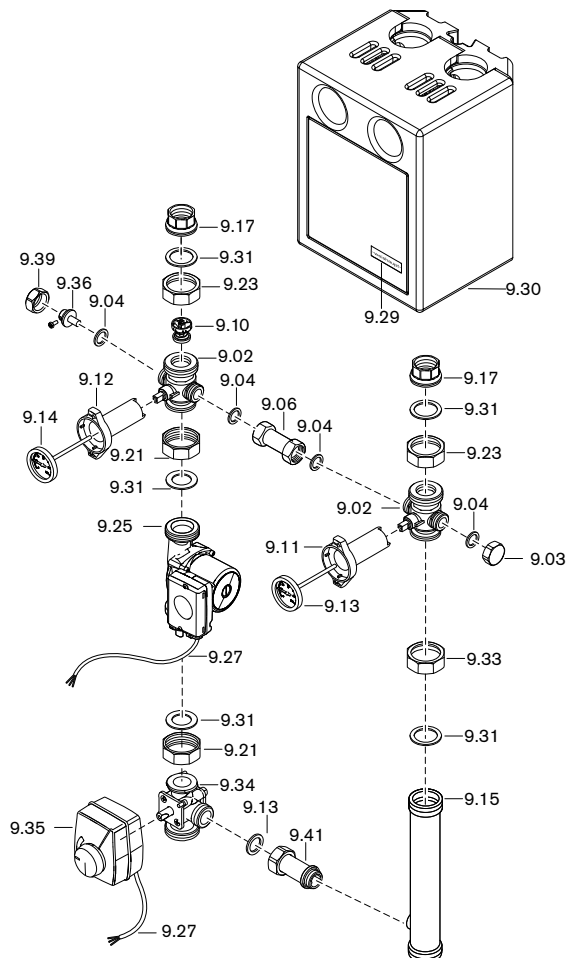
Mischergruppe / mixer assembly / groupes de mélange NW32
