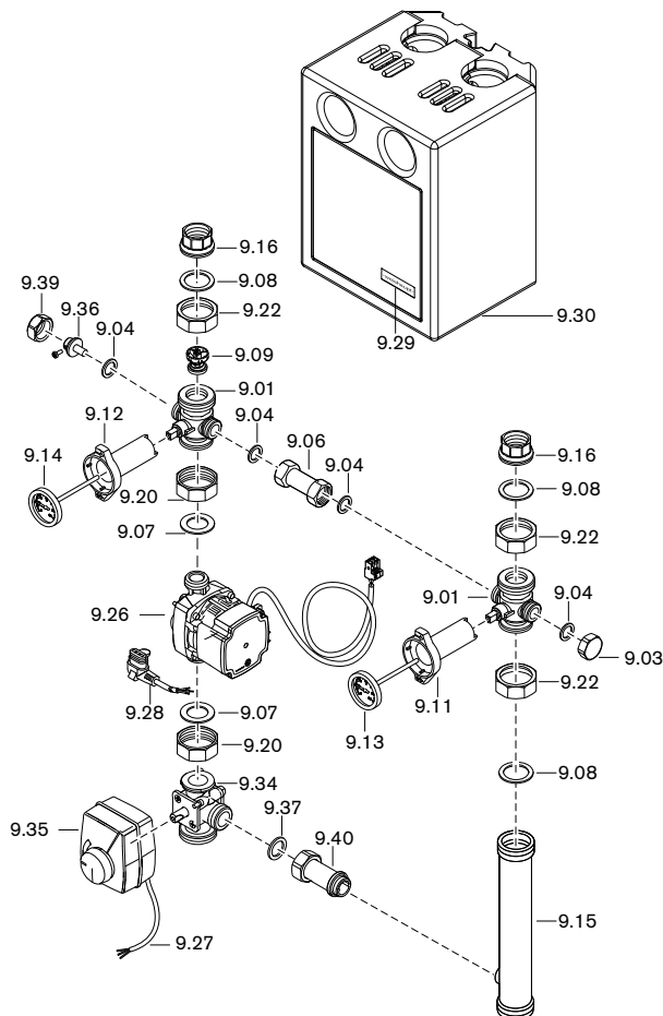
Mischergruppe / mixer assembly / groupes de mélange NW25
