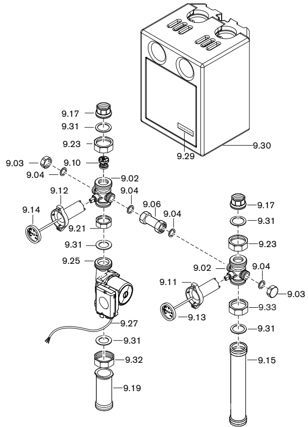
Mischergruppe / mixer assembly / groupes de mélange NW32
